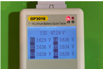
fig. 1E – Individual cell values.
